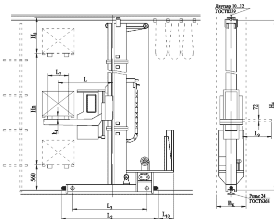
Рис.1 Общий вид электроштабелера высотного стеллажного ТС-10М
